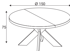
Dining table D150(250max)
