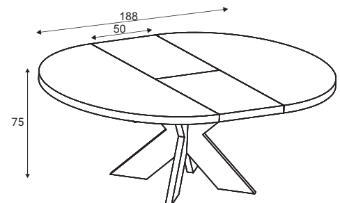
Dining table D150(200)
